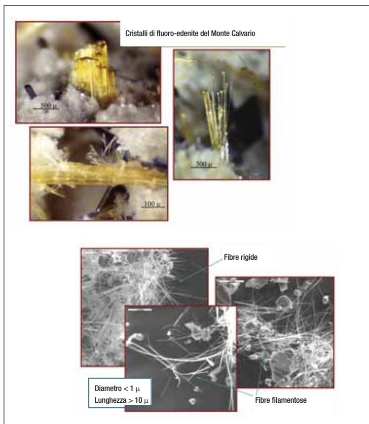
Figura 15. - In alto: cristalli di fluoro-edenite prelevati dal Monte Calvario osservati in microscopia ottica. In basso: fibre anfiboliche di fluoro-edenite osservate in microscopia elettronica.
