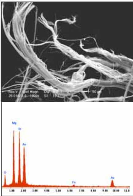
Figura 3. - Fibre di amianto crisotilo osservate in microscopia elettronica a scansione (in alto) e spettro elementare tipico delle stesse ottenuto mediante microanalisi a raggi X a dispersione di energia (in basso).
